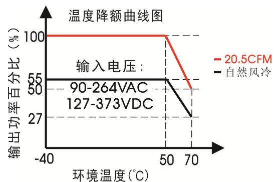
LOF350-20B15-C(满载 325W 带 20.5CFM 风扇)
