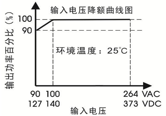
LOF350-20Bxx-C 输入电压降额
