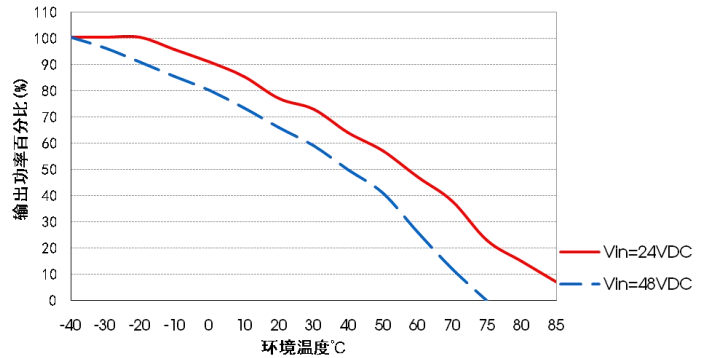
URF4812/24/48QB-200WFR3 温度降额曲线
