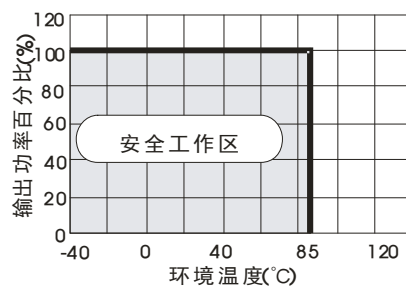
温度曲线图
