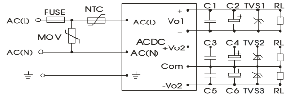
图 4: LH20-10C 系列(三路)典型应用电路
