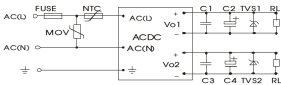
图 3: LH20-10D 系列(双隔离双路)典型应用电路
