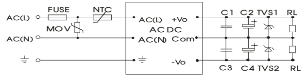
图 2: LH20-10A 系列(正负双路)典型应用电路
