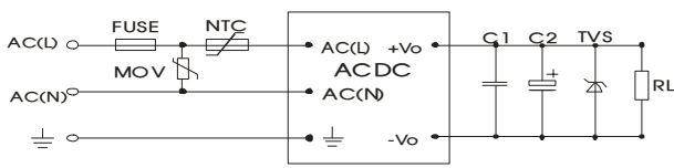
图 1: LH20(25)-10B 系列(单路)典型应用电路
