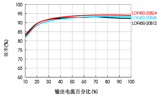
效率Vs输出负载 (Vin=230VAC)
