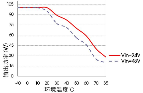
URF4805QB-100WFR3 温度降额曲线
